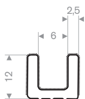
219.01.108 EPDM gevlokt
