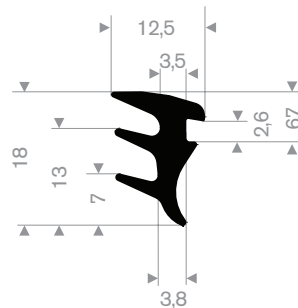
216.03.557 EPDM 65° Shore zwart
