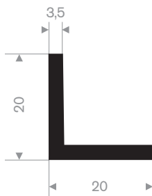
216.52.020 EPDM 70° Shore zwart
