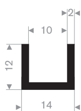
211.01.210 EPDM 70° Shore zwart
