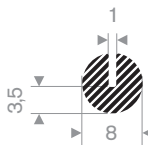
221.01.108 EPDM 15° Shore zwart
