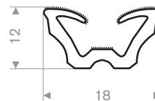
219.01.204 EPDM gevlokt
