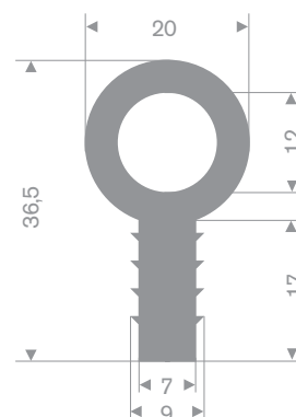
216.03.101 EPDM 70° Shore grijs
