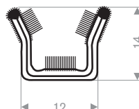
219.01.022 EPDM + textiel
