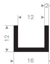
211.01.212 EPDM 70° Shore zwart
