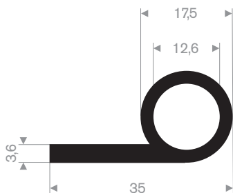
214.00.815 EPDM 70° Shore zwart
