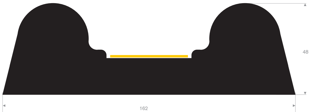
215.01.210 EPDM 70° Shore zwart lengte 1 meter
