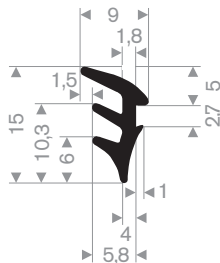
216.03.551 EPDM 65° Shore zwart
