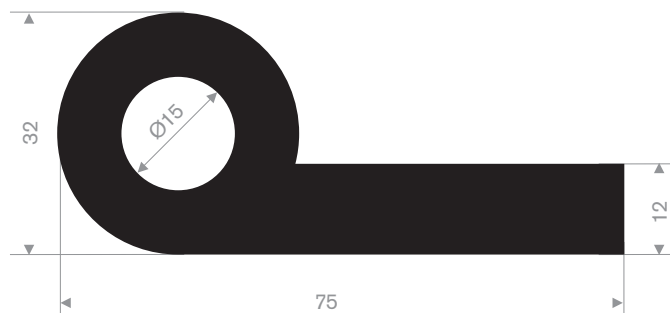
214.00.866 EPDM 70° Shore zwart
