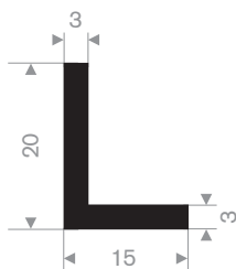
216.52.015 EPDM 70° Shore zwart
