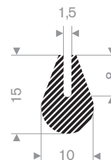
221.00.110 EPDM 15° Shore zwart
