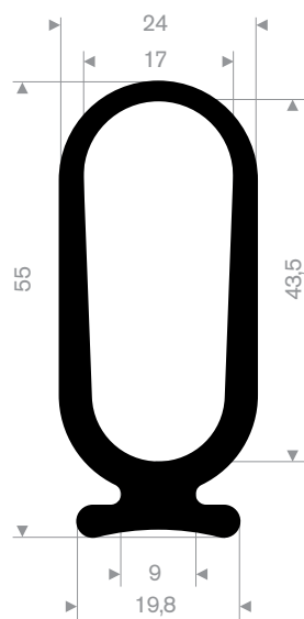
216.01.125 EPDM 70° Shore
