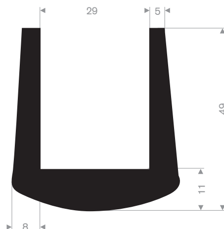
211.05.511 EPDM 70° Shore zwart
