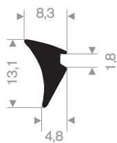
216.03.633 EPDM 70° Shore zwart
