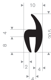
212.00.048 EPDM 70° Shore zwart
