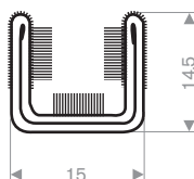
219.01.021 EPDM + textiel
