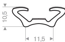
219.01.201 EPDM gevlokt
