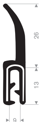
245.00.875 pvc + volrubber klembereik 1,5-4 mm
